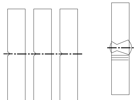
Zóna tepelně ovlivněná svarem
