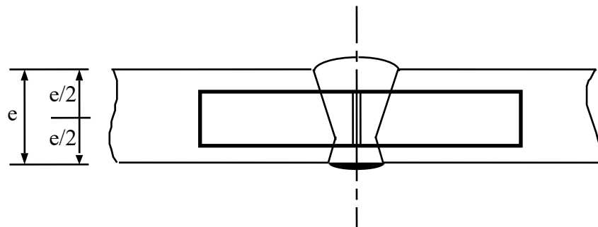
Střed svaru
