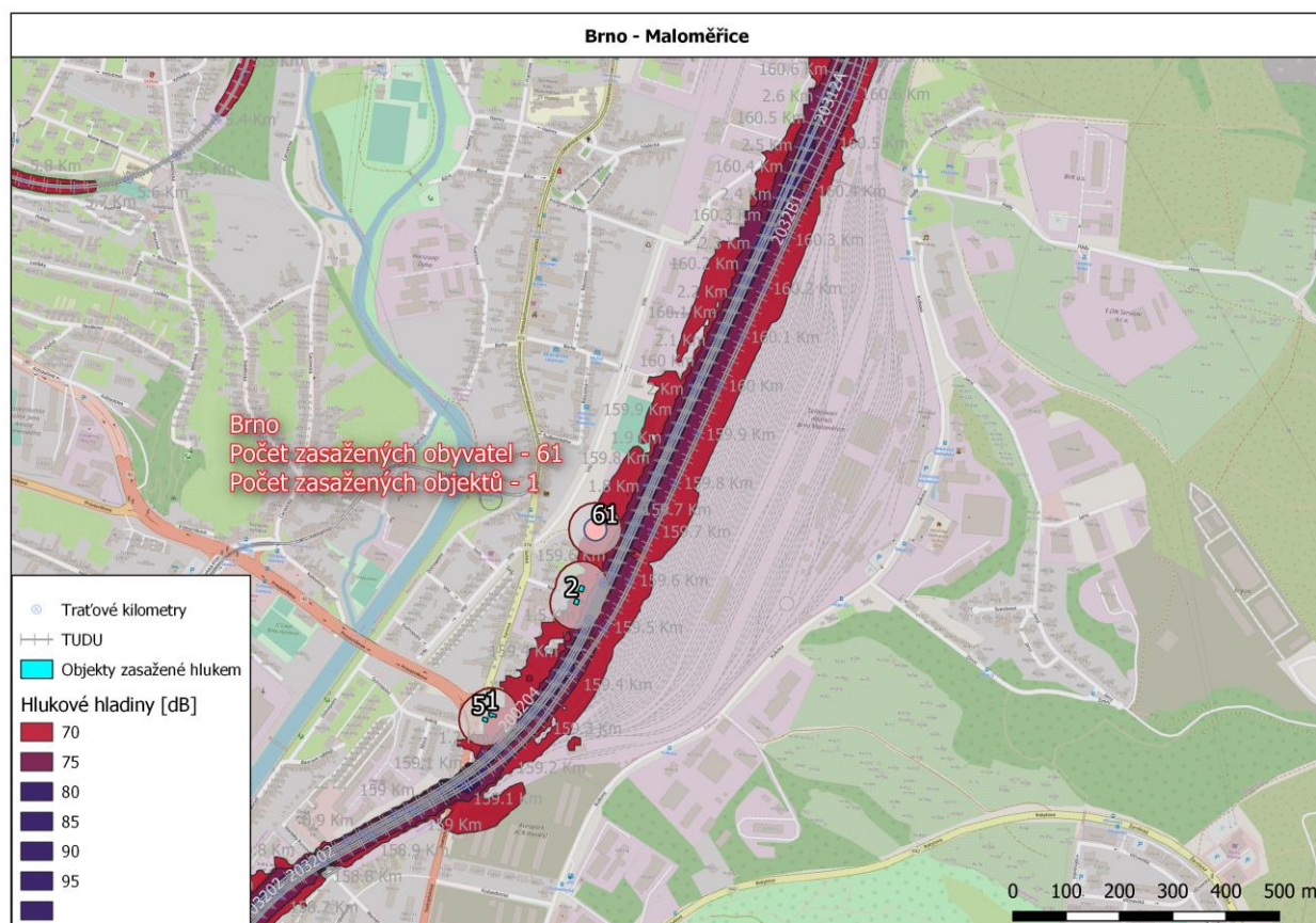
Obrázek 17 Hotspot Brno – Maloměřice
