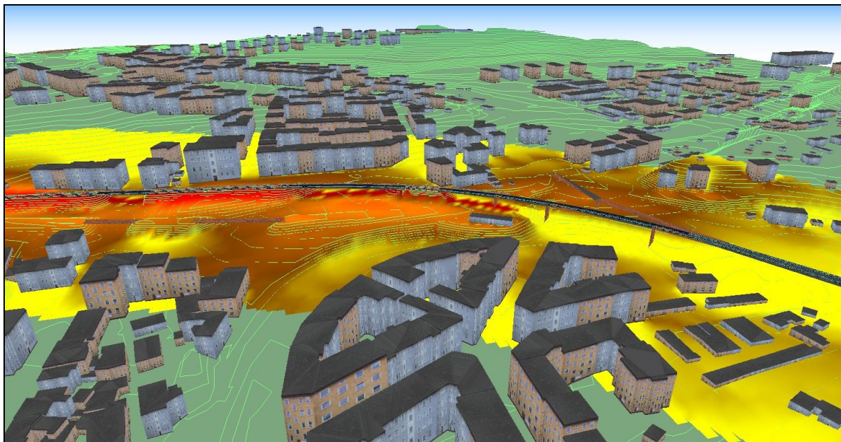
Obrázek 10 Příklad 3D zobrazení aktualizace dat v ukazateli Ln u konkrétního hot spotu (Praha – Libeň)
