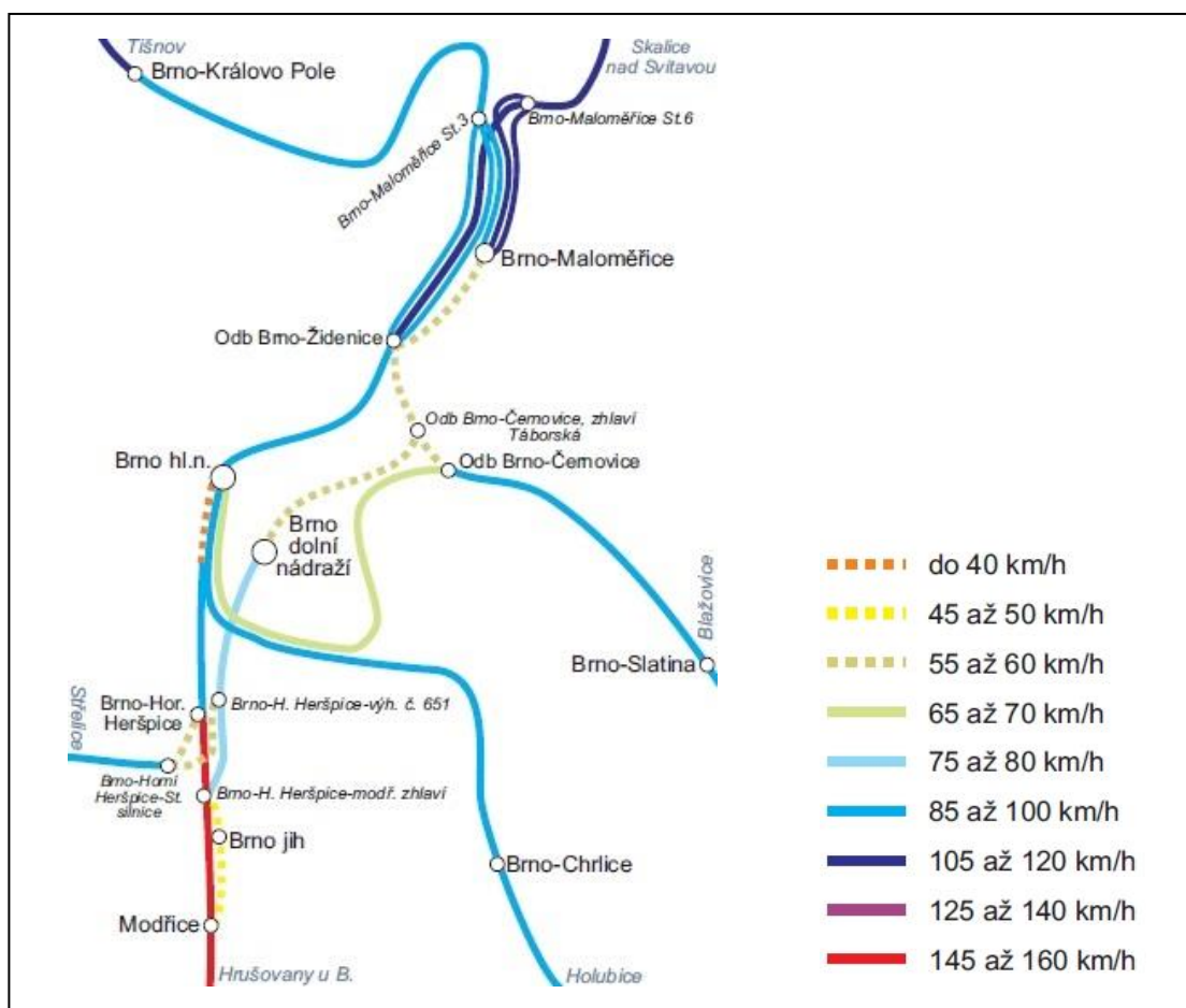
Obrázek 7 Maximální povolené traťové rychlosti v železniční síti širšího okolí Brna
