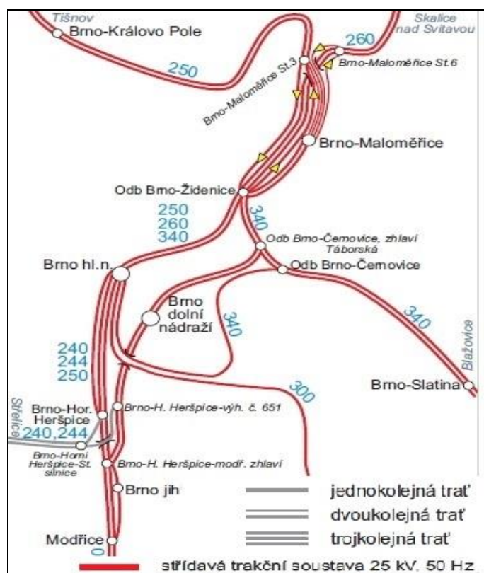
Obrázek 6 Počty kolejí, systémy trakčních proudových soustav a označení dle KJŘ
