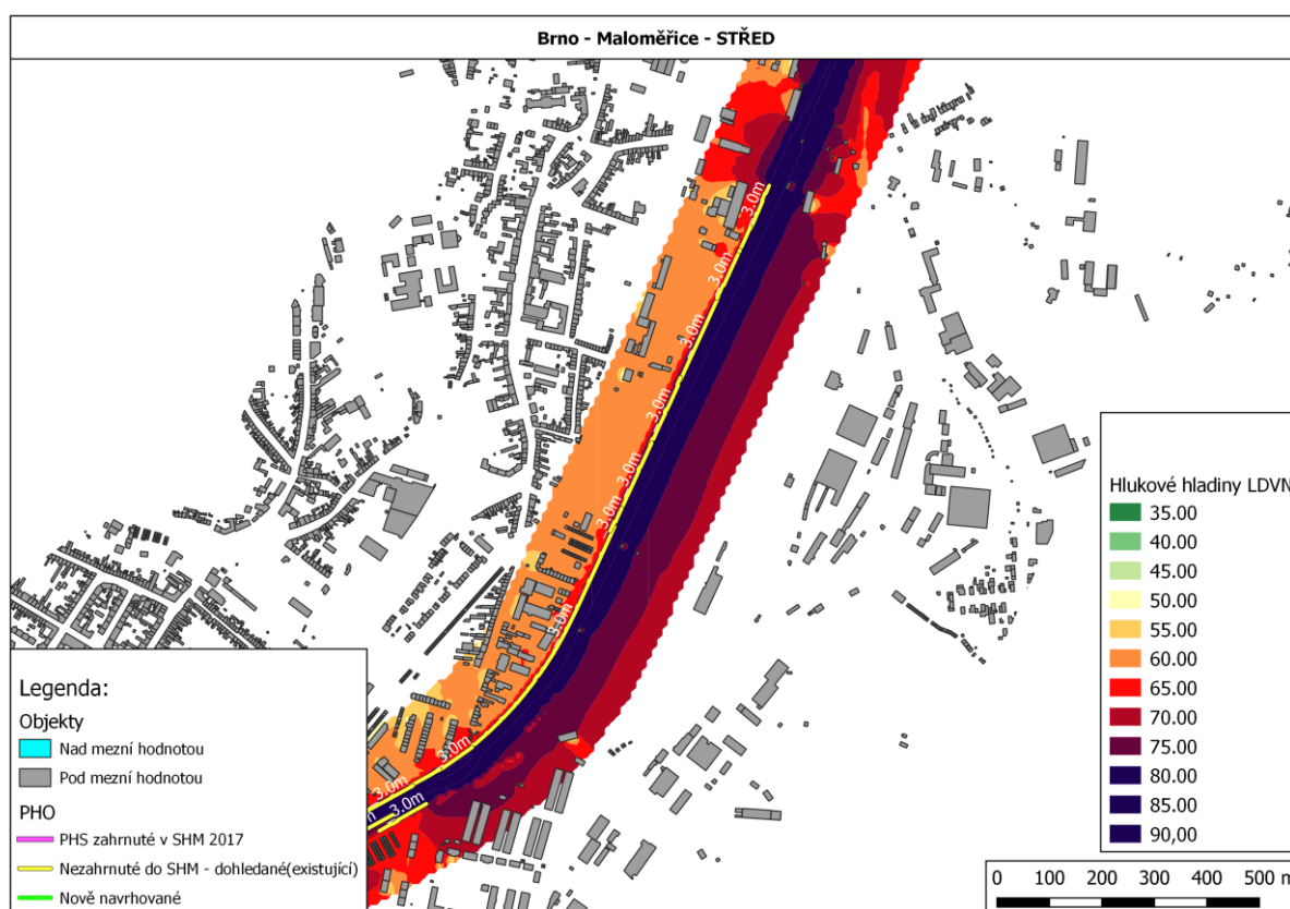
Obrázek 18 Protihluková opatření - Brno – Maloměřice
