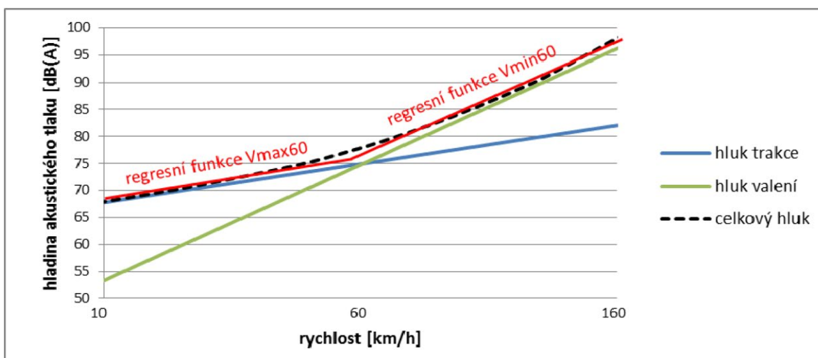
Obrázek 5 - Závislost hladiny akustického tlaku na rychlosti s regresními funkcemi (Týfa, Ládyš a kol. 2013)
