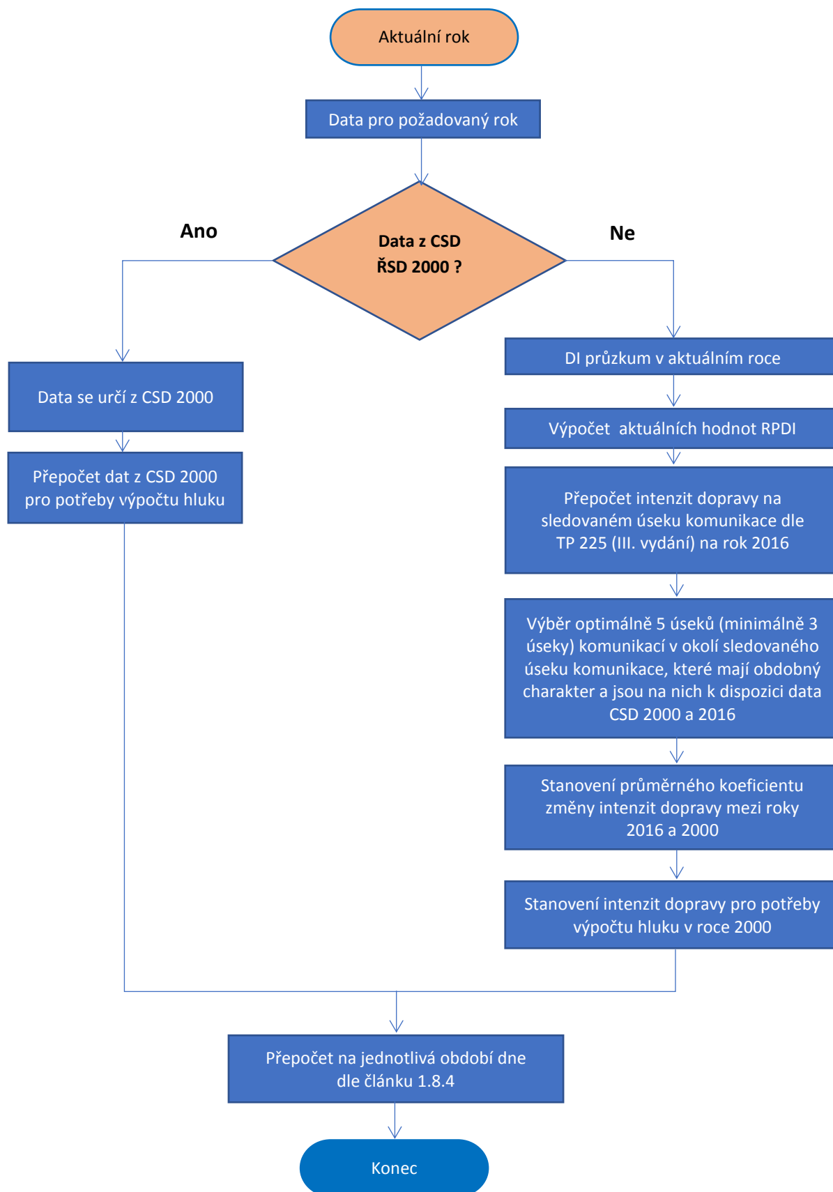
Obr. B.1: Postupový diagram zpětného přepočtu intenzit dopravy pro rok 2000
