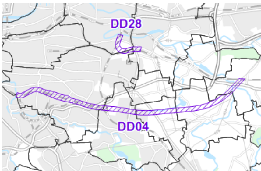
Obr. 14 Jahodnická spojka – výřez z výkresu I.1 grafické části DÚRP VRT PRAHA
