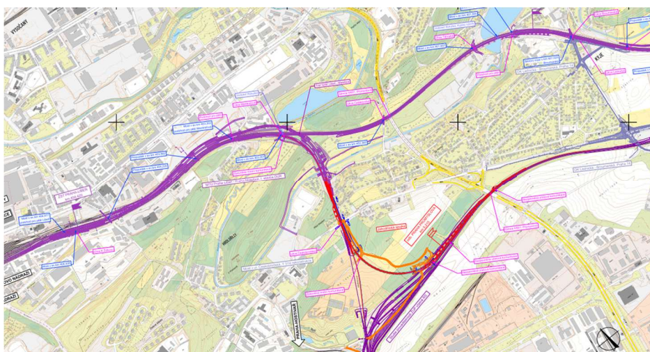
Obr. 15 Jahodnická spojka – detail technického řešení
