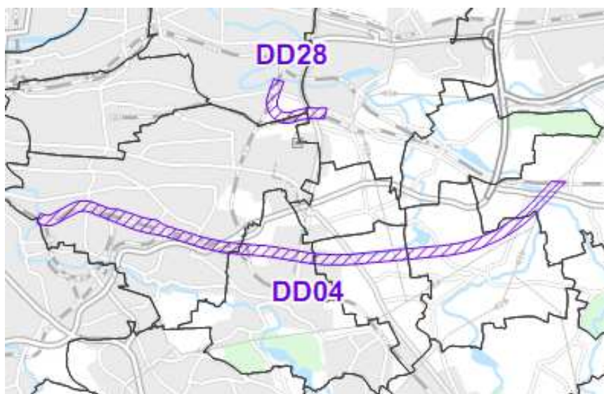
Obr. 14 Jahodnická spojka – výřez z výkresu I.1 grafické části DÚRP VRT PRAHA
