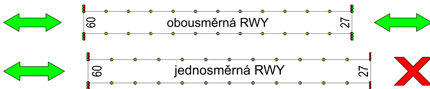
Obr. 5-4 Použití prahových a koncových dráhových návěstidel u obousměrných i jednosměrných RWY.
