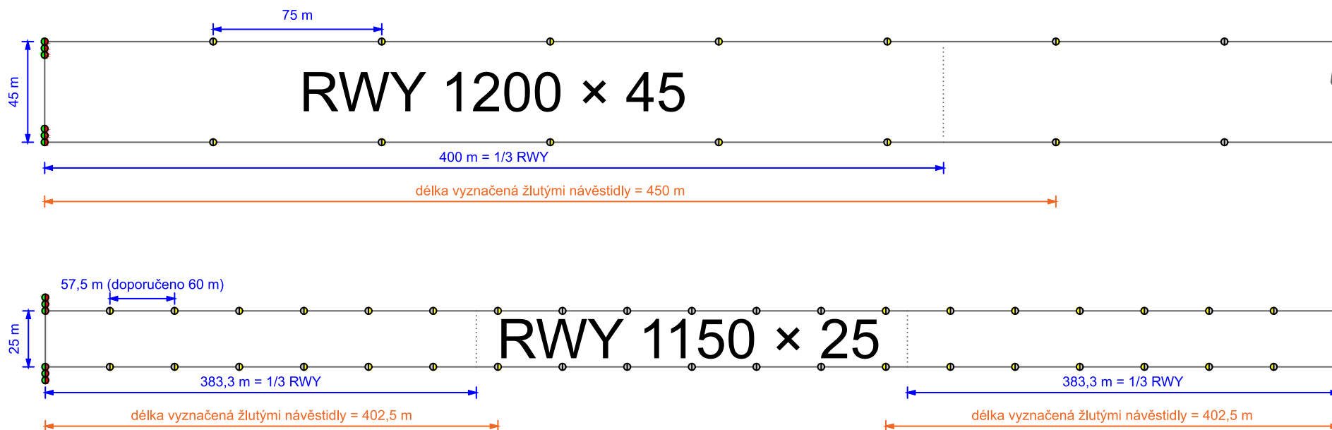
Obr. 5-2 Příklady rozmístění postranních návěstidel RWY tam, kde je úseku vyznačený žlutými návěstidly delší než 1/3 délky RWY. (Obrázek je totožný s Obr. 5-2)
