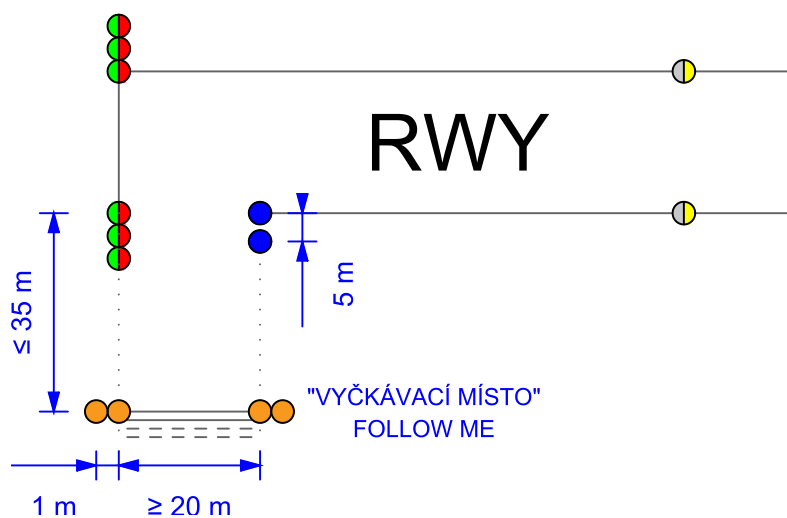
Obr. A-19 Zátáčka/zalomení TWY pod úhlem 45°-90°
