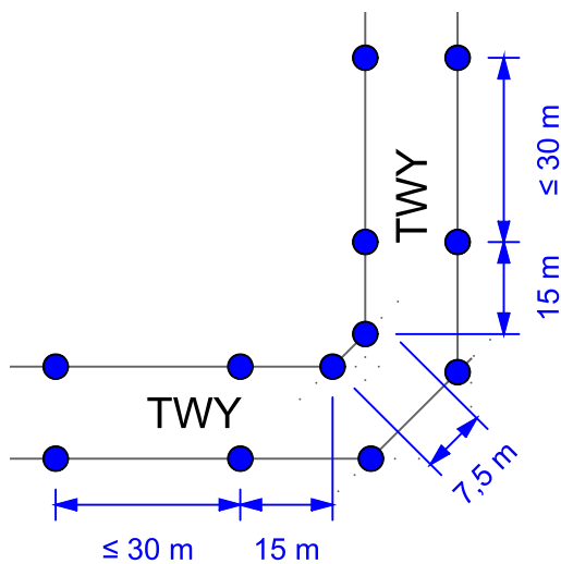
Obr. A-19 Zátáčka/zalomení TWY pod úhlem 45^{\circ} - 90^{\circ}
