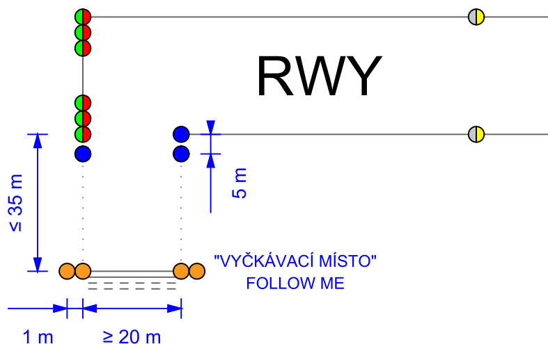
Obr. A-18 Zátáčka/zalomení TWY pod úhlem 10°-45°
