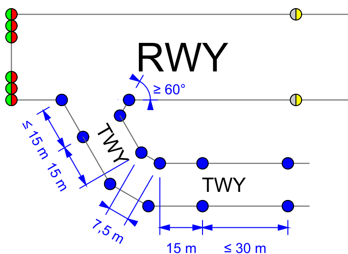
Obr. A-12 Šikmé napojení ( 90^\circ\text{-}60^\circ ) paralelní TWY na RWY mimo její konec s rozšířením v oblasti napojení
