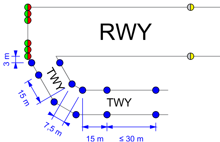
Obr. A-11 Šikmé napojení ( 90^\circ\text{-}60^\circ ) paralelní TWY na RWY na jejím konci s vnitřními polopříčkami THREND
