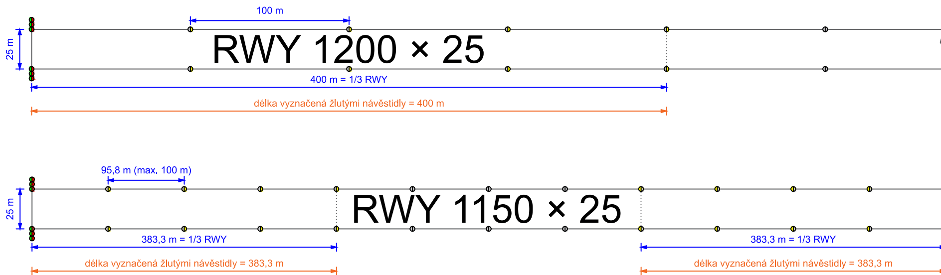
Obr. B-1 Příklad rozmištění postranních návěstidel RWY tam, kde je úseku vyznačený žlutými návěstidly roven 1/3 délky RWY. (Obrázek je totožný s Obr. 5-1)
