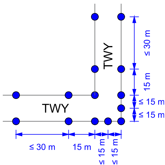
Obr. A-20 Zátáčka/zalomení TWY pod úhlem 90^{\circ}
