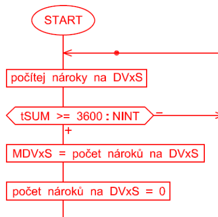
Obr. 14 VD 101 – algoritmus součtu nároků na vybraném detektoru pro rozhodování o výběru a ukončení „fáze blikající žlutá“, běží při všech programech a způsobech řízení
