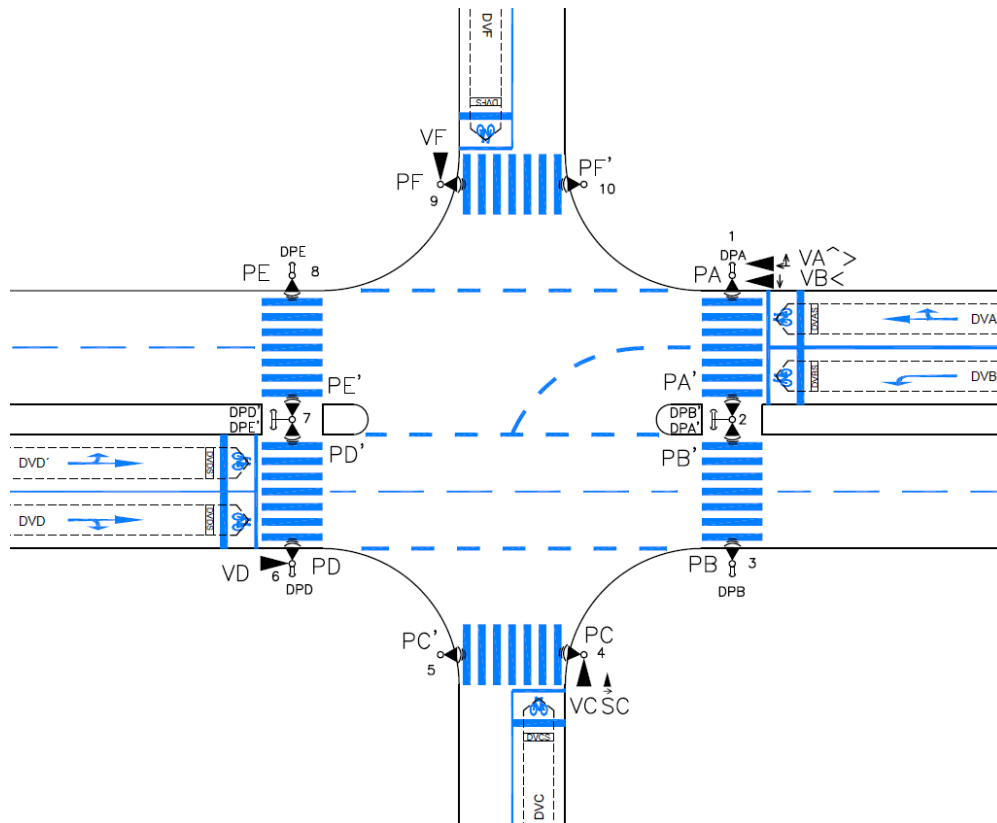
Obr. 6 Situační schéma křižovatky [9]
