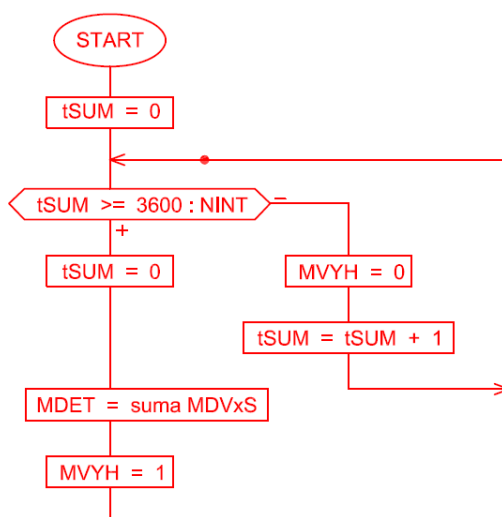
Obr. 15 VD 102 – algoritmus součtu nároků na všech vybraných detektorech pro rozhodování o výběru a ukončování „fáze blikající žlutá“, běží při všech programech a způsobech řízení
