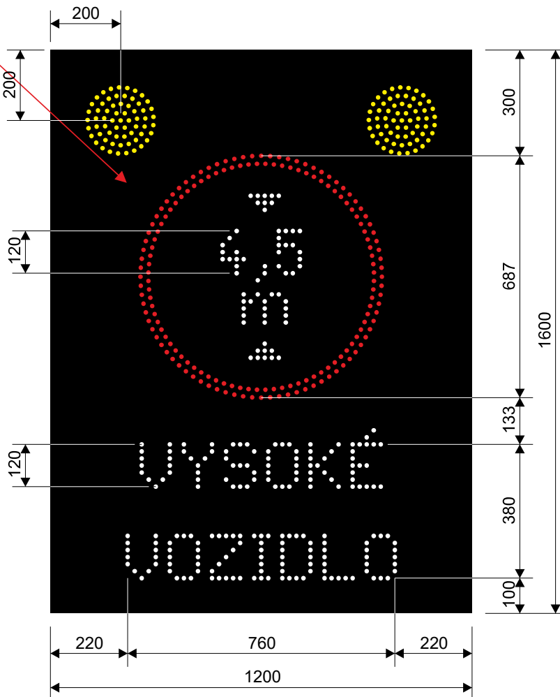
Tabulka roztečí
