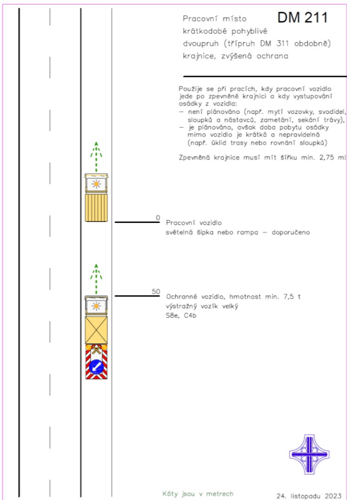
Schema DM 211 Využití při montáži a demontáži PDZ
