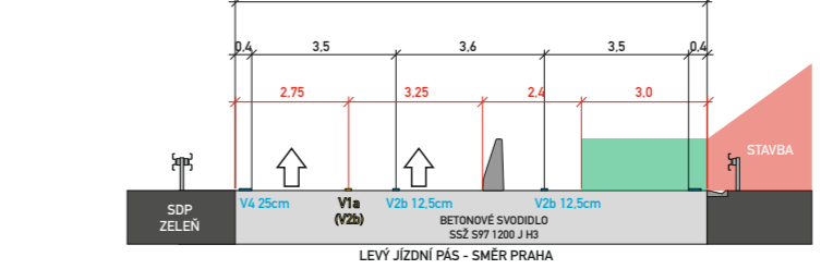
Příčný řez profilem dátnice D4 Pravý jízdní pás v km 43.519
