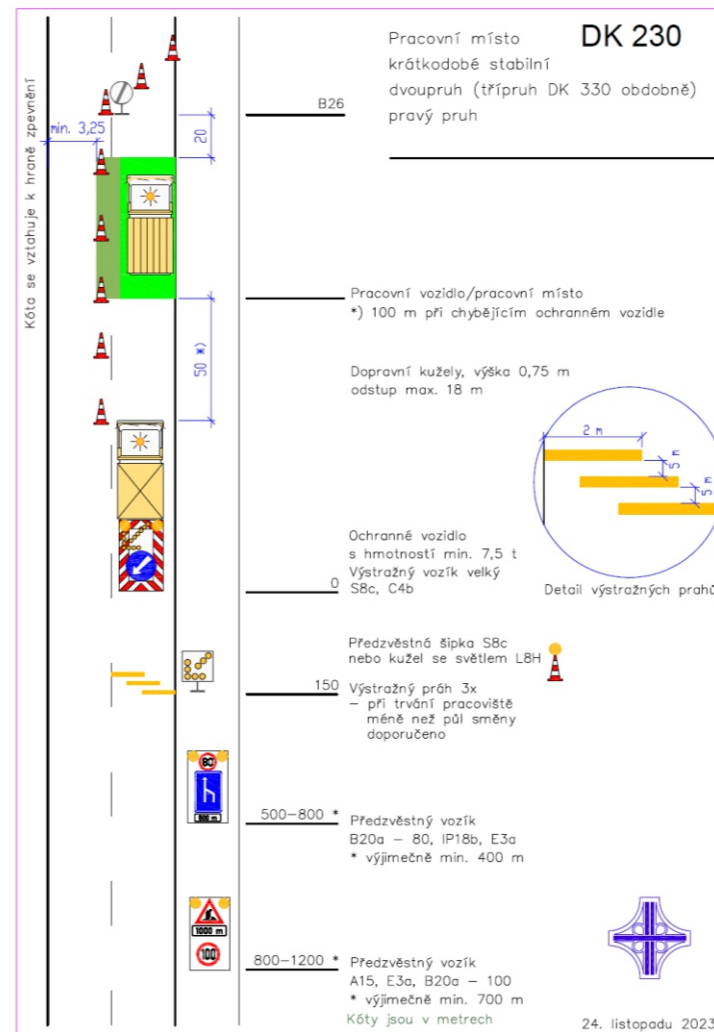
Schema DK 230 Využití při montáži a demontáži stěny z betonových svodidel
