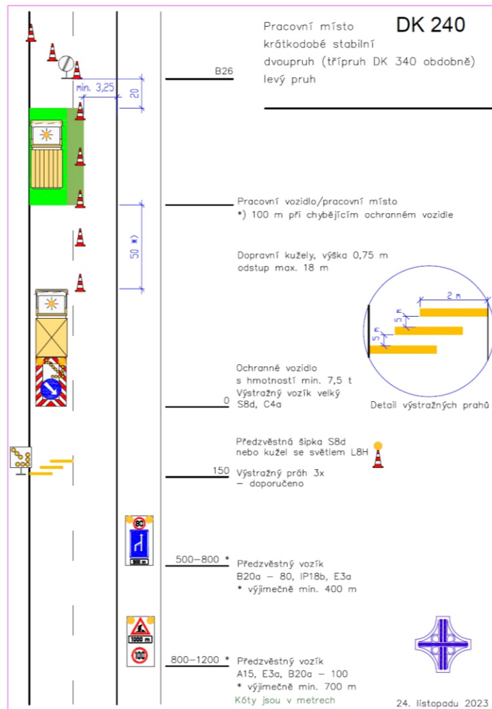
Schema DK 240 Využití při instalaci a odstranění přechodného VZD
