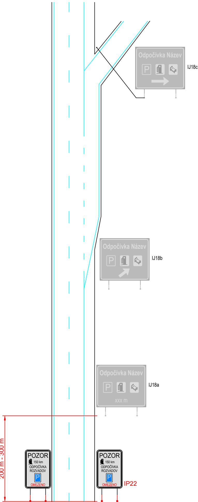
VZOROVÉ SCHÉMA UMÍSTĚNÍ DZ IP22
