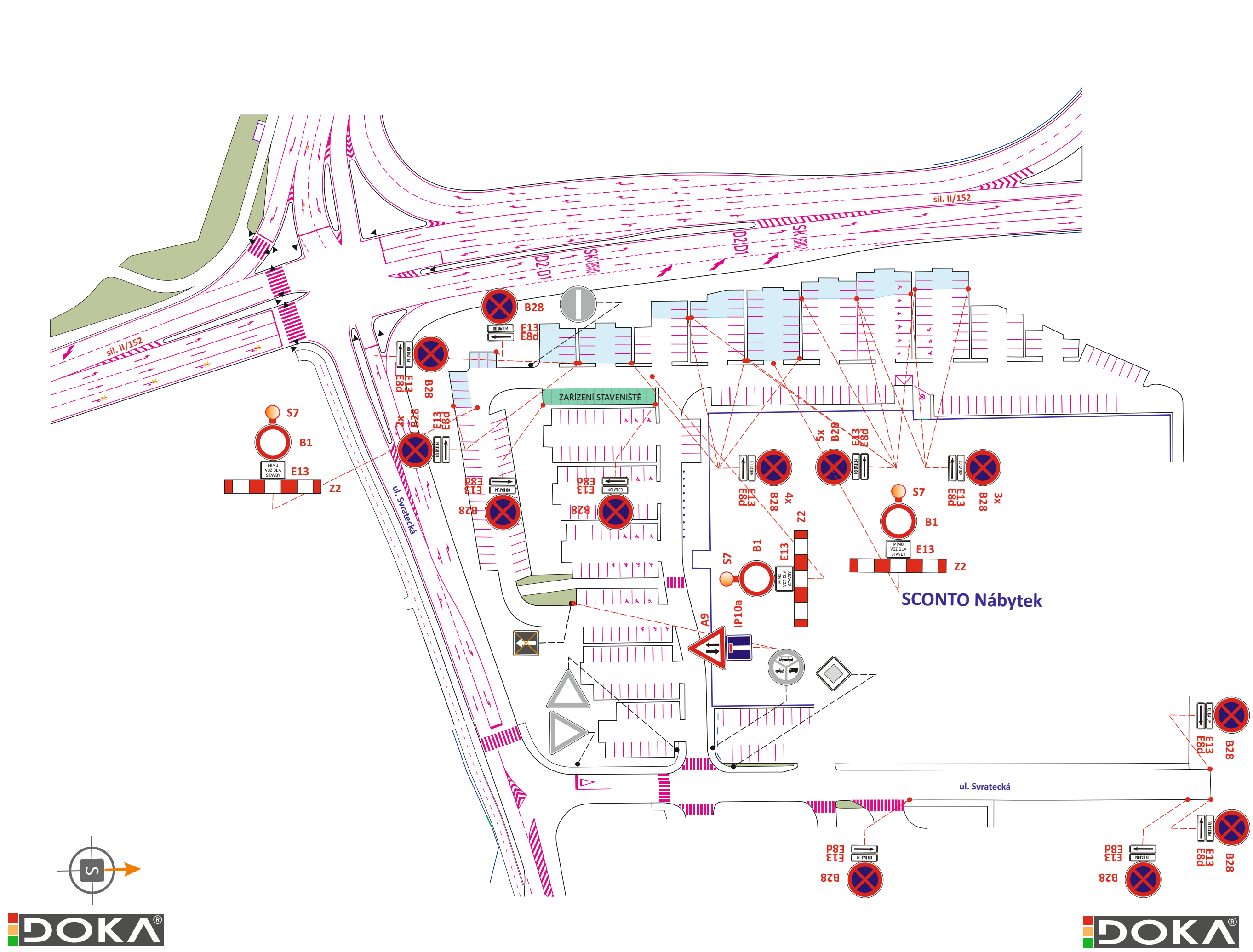
PARKOVIŠTĚ SCENTO NÁBYTEK - ZÁBORY V MÍSTĚ PARKOVACÍCH STÁNÍ
