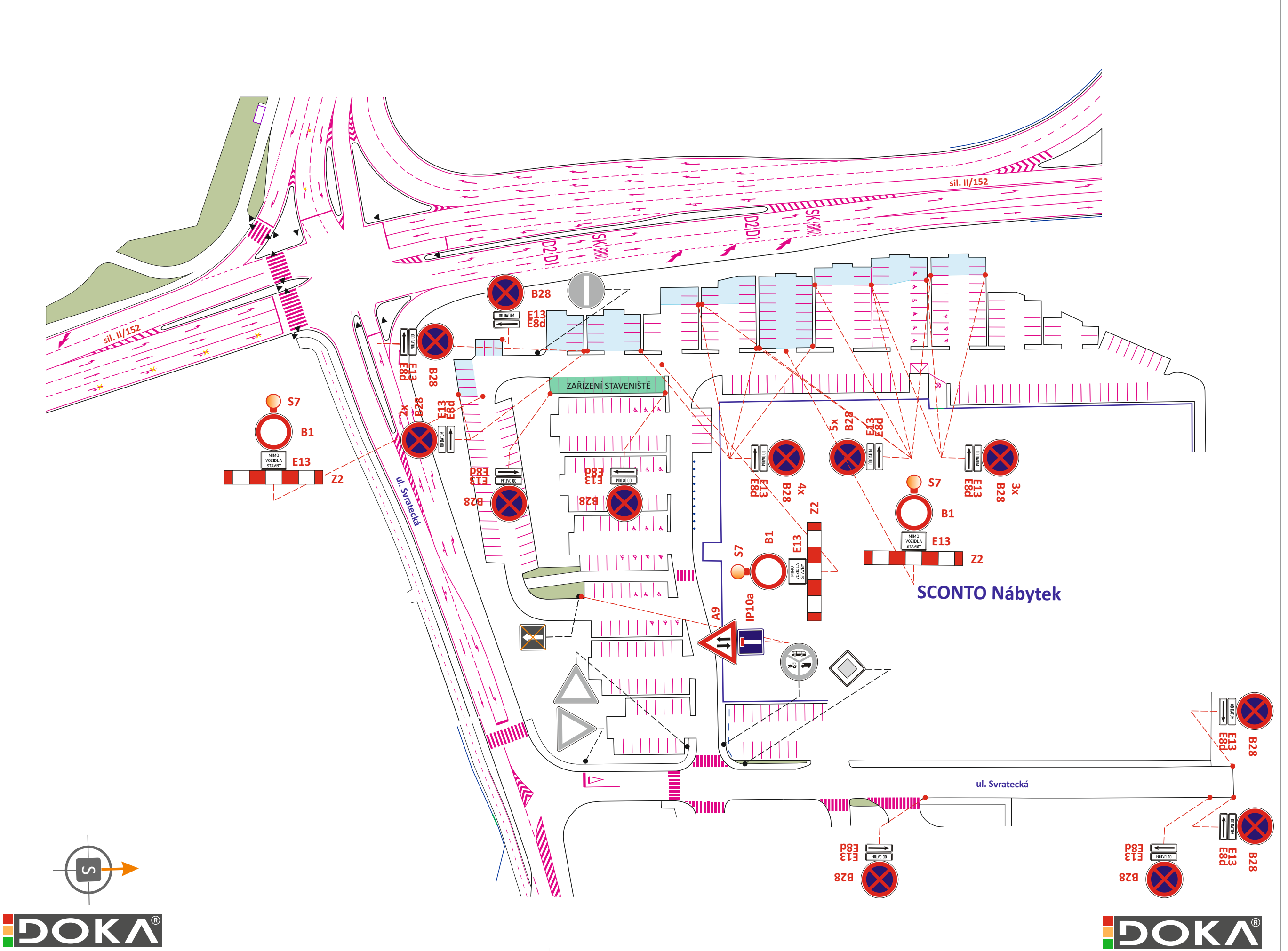
PARKOVIŠTĚ SCONTO NÁBYTEK - ZÁBORY V MÍSTĚ PARKOVACÍCH STÁNÍ
