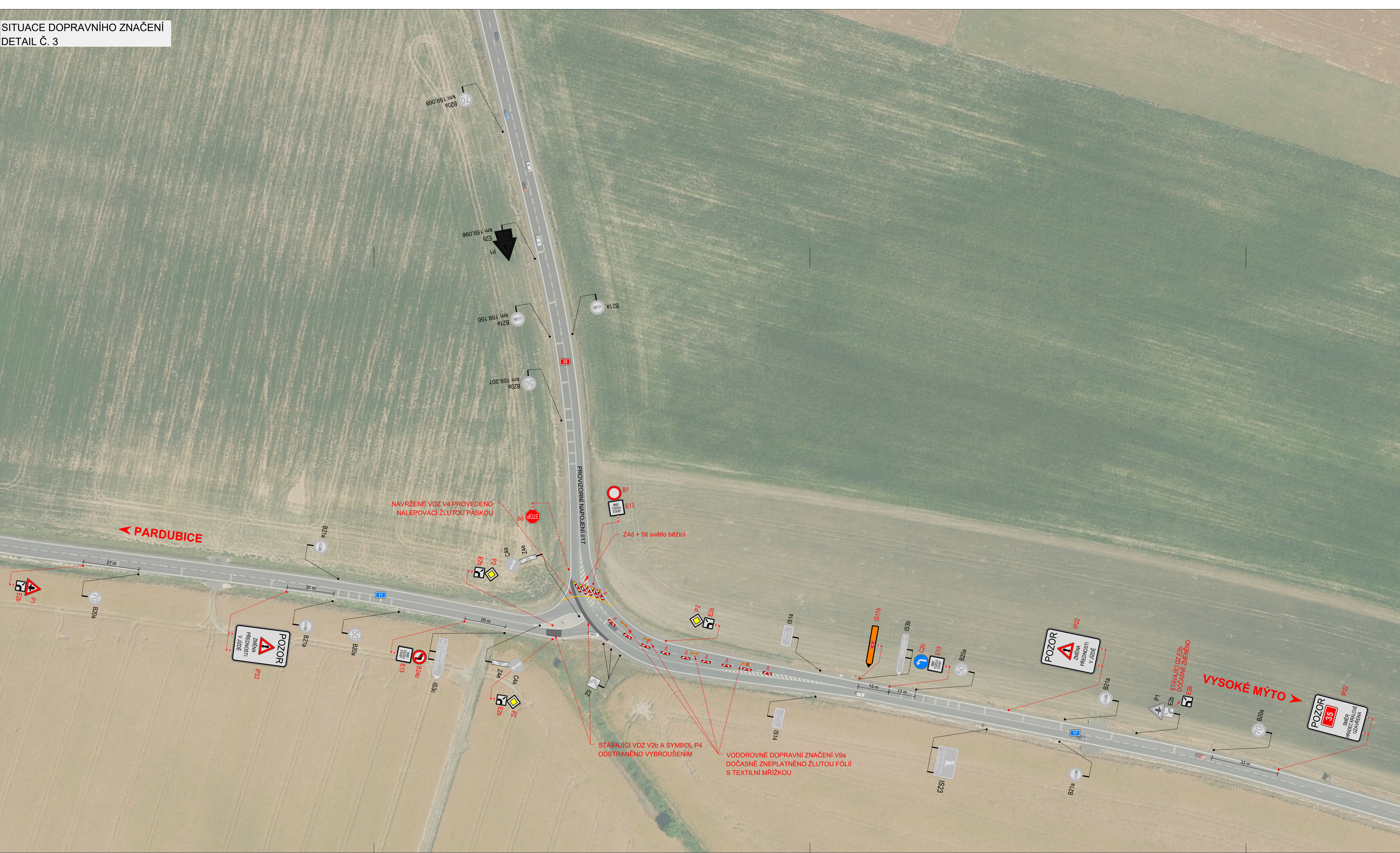
SITUACE DOPRAVNÍHO ZNAČENÍ DETAIL Č. 2
