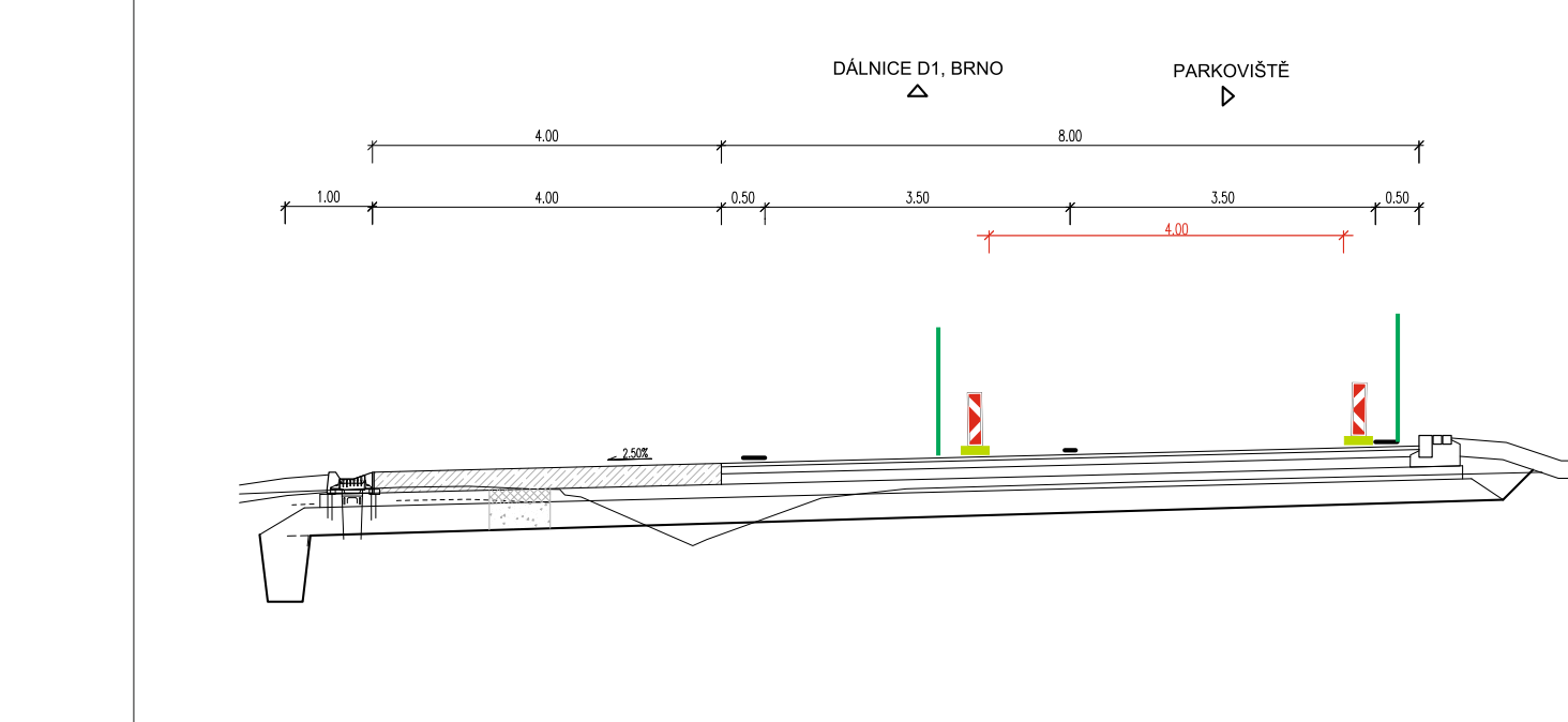
VZOROVÝ PŘÍČNÝ ŘEZ A - A'
