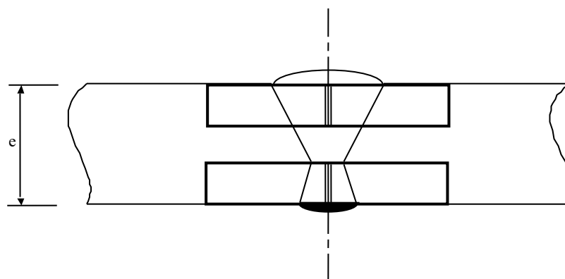
Střed svaru
