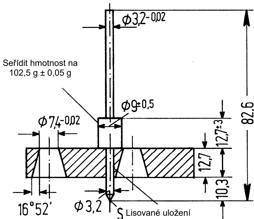
Penetrometr
